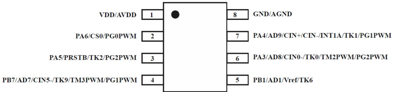
SZY8T663系列SOP8
