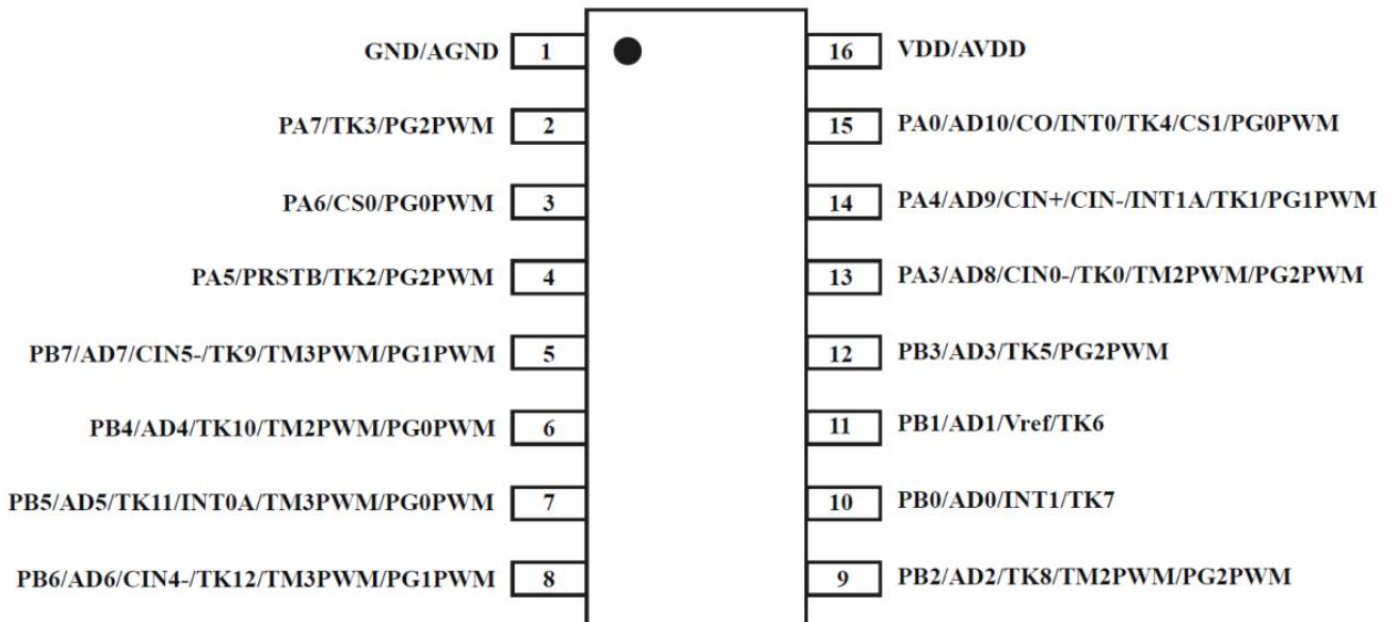
SZY8T663系列SOP16
