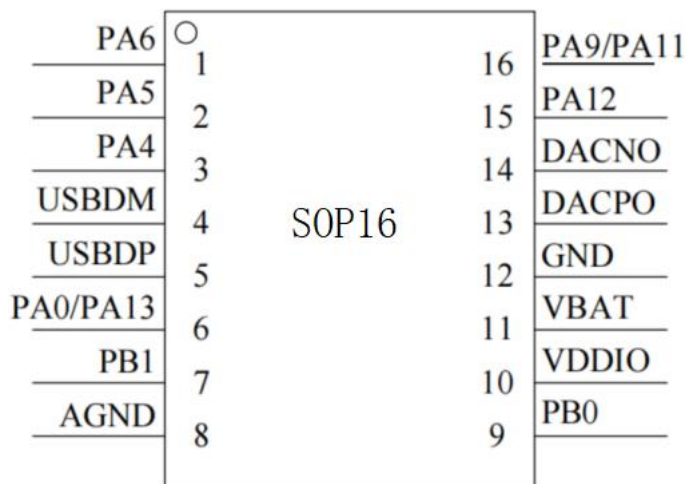
图2-1 SZY42F-SOP16封装图
