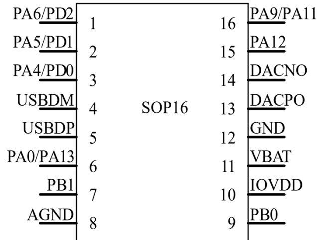
图2-1 SZY42F-SOP16封装图
