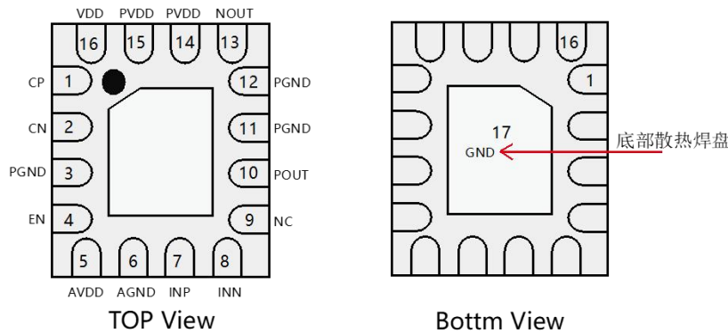
图 2 芯片顶视图和底视图
