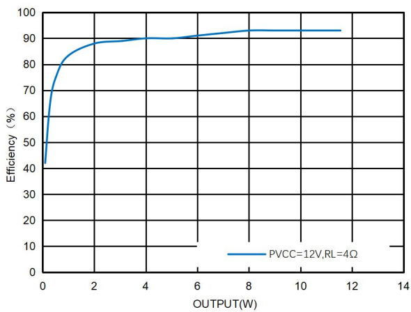
图24. 效率曲线
