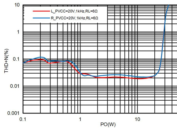
图17. 20V供电6Ω负载THD+N曲线BTL
