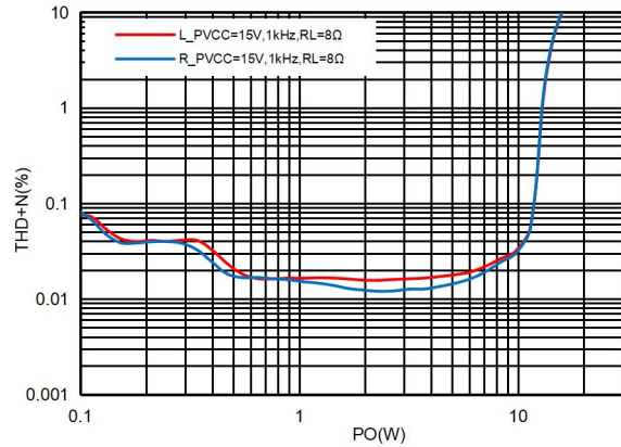
图19. 15V供电8Ω负载THD+N曲线BTL
