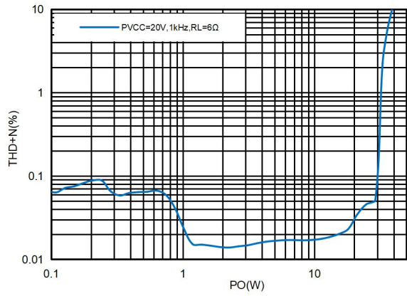
图32. 20V供电6Ω负载THD+N曲线PBTL
