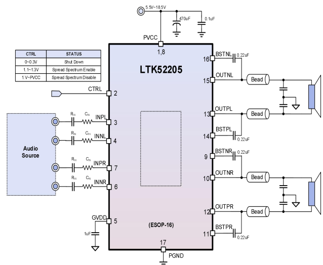
图1. LTK52205 简化应用原理图
