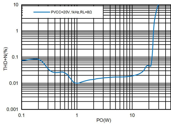
图36. 20V供电8Ω负载THD+N曲线PBTL
