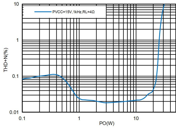
图27. 15V供电4Ω负载THD+N曲线PBTL
