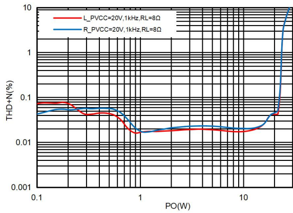
图21 20V供电8Ω负载THD+N曲线BTL
