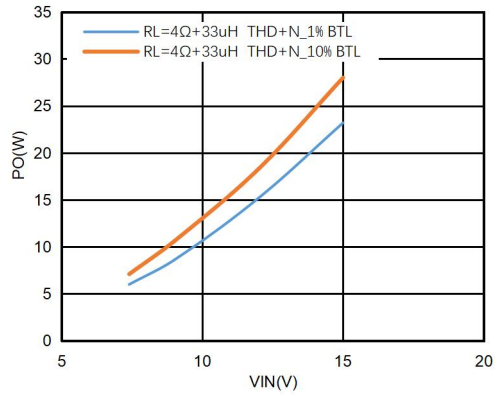
图8. 4Ω负载下不同电源电压的THD+N
