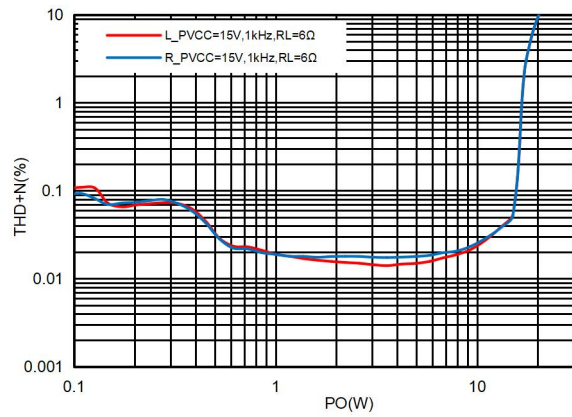
图15. 15V供电6Ω负载THD+N曲线BTL
