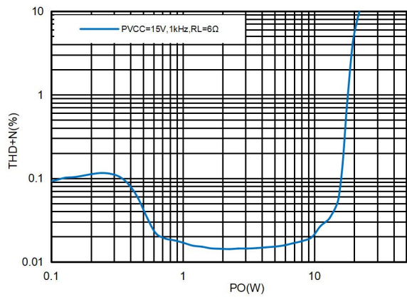
图30. 15V供电6Ω负载THD+N曲线PBTL
