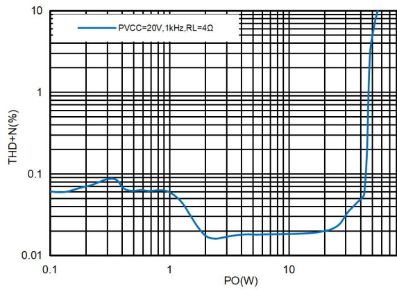
图29. 20V供电4Ω负载THD+N曲线PBTL
