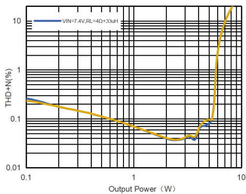
图12. 7.4V电压、4Ω负载输出功率和THD+N
