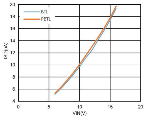
图10. 不同电源电压下关断电流
