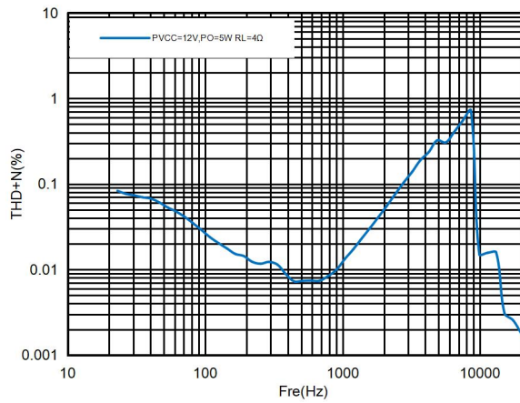
图25. 频率失真曲线
