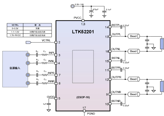
图1. LTK52201 简化应用原理图
